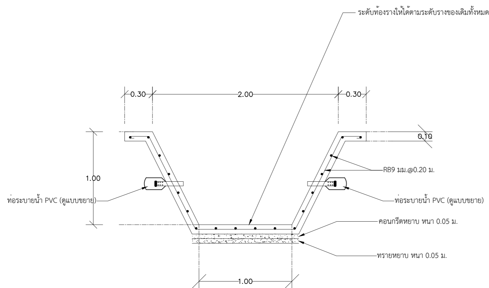
ขยายรางระบายน้ำคอนกรีตรูปตัว U
