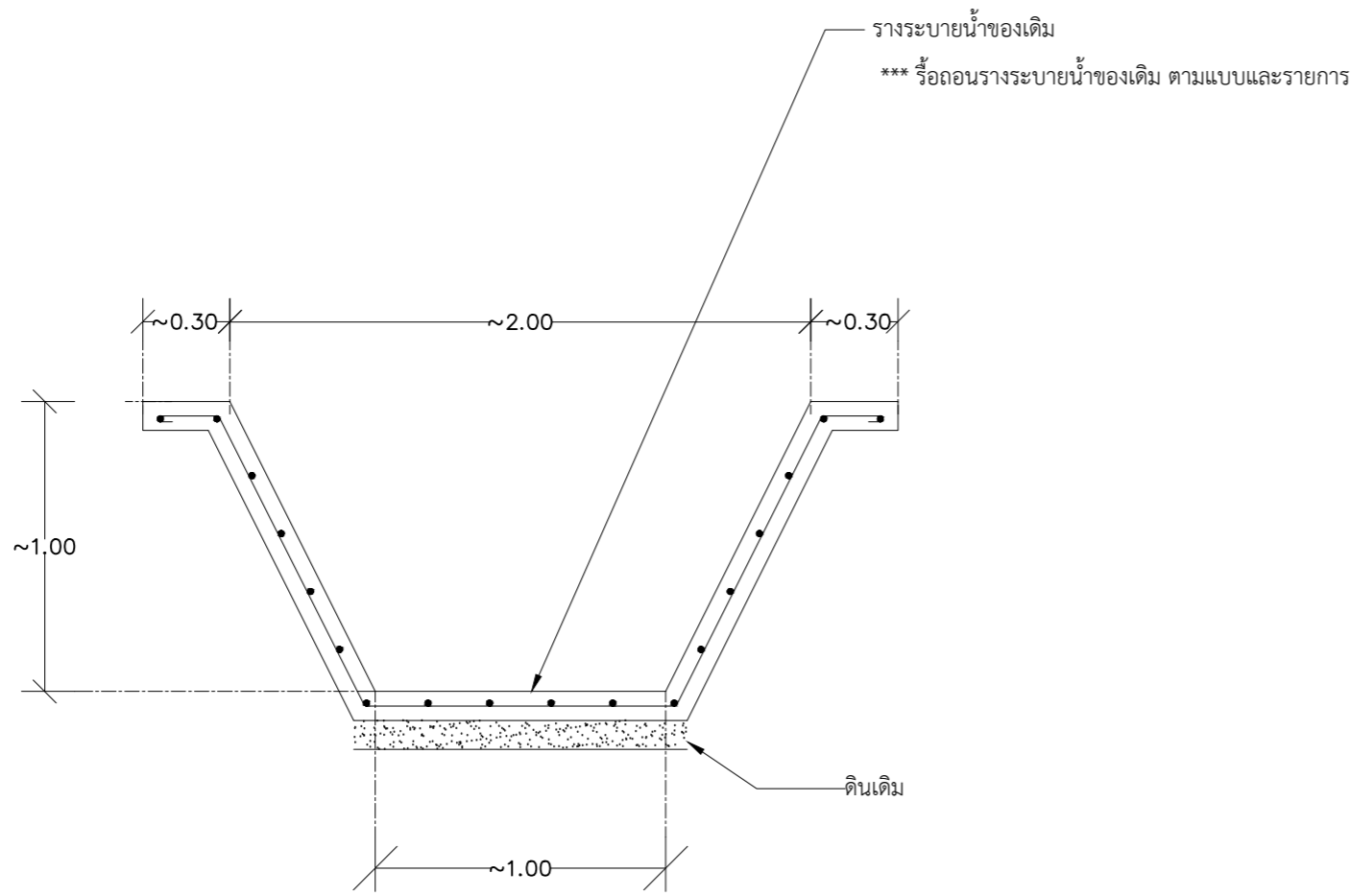
แสดงรูปตัดรางระบายน้ำ ของเดิม
