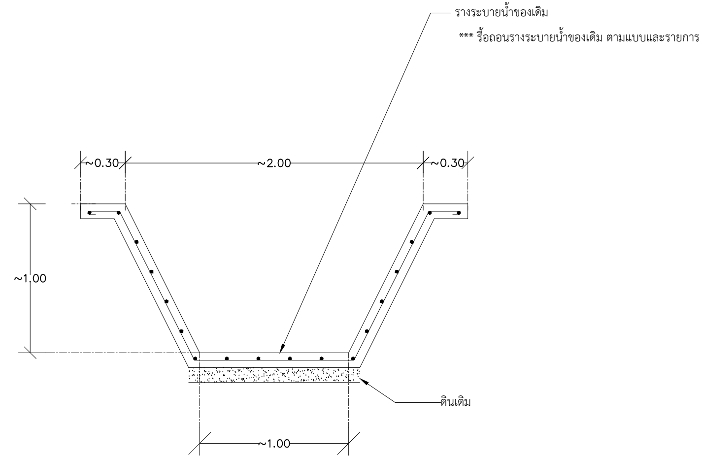
แสดงรูปตัดรางระบายน้ำ ของเดิม
